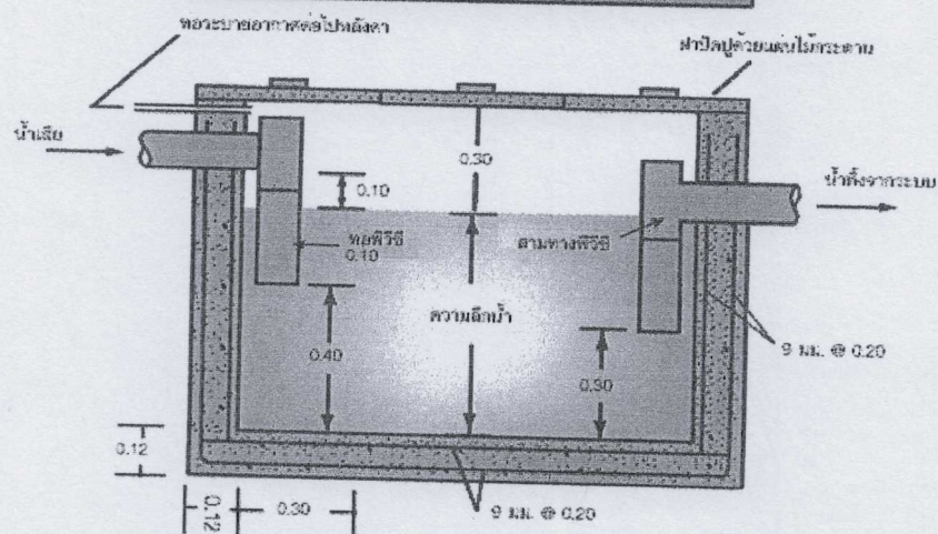
บ่อดักไขมันแบบสร้างในที่สำหรับอาคารขนาดใหญ่
